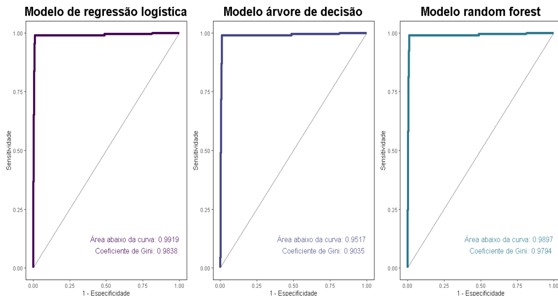
Figura 3: Comparativo das medidas de desempenho dos modelos de classificação regressão logística binária, árvore de decisão e random forest Fonte: Dados originais da pesquisa
